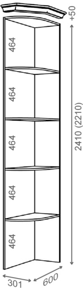
Карниз на угол 600
